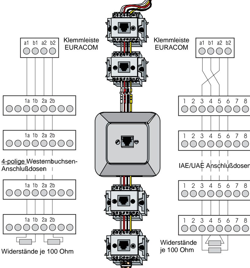
Verdrahtung des internen ISDN-Busses
