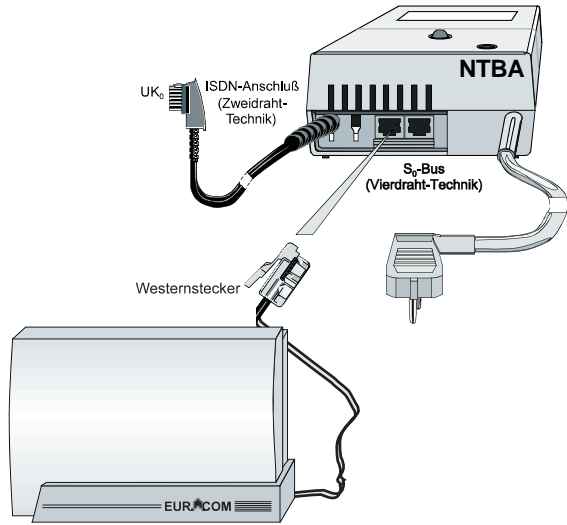
Anschluß der Tk-Anlage an den NTBA
