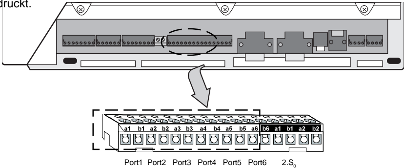
Steckerleistenbelegung für den Anschluß der 6 analogen Teilnehmer an eine EURACOM 26x
