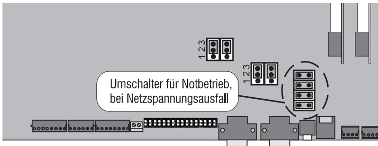
Ansicht des Tk-Anlagen-Innenraumes, mit Umschalter für Notbetriebsfunktion (gekennzeichnete Darstellung vergrößert)
