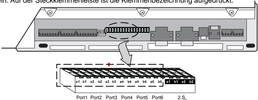
Steckerleistenbelegung für den Anschluß der 6 analogen Teilnehmer an eine EURACOM 26xF
