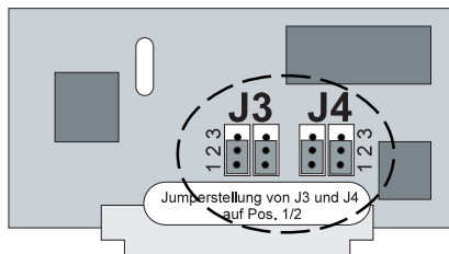
Jumper-Position für den Betrieb als interner ISDN-Bus mit Speisung
