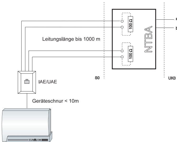
ISDN-Anlagenanschluß – Punkt-zu-Punktanschluß
