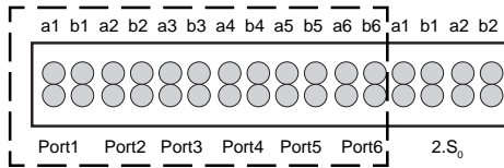
Steckerleistenbelegung für den Anschluß der 6 analogen Teilnehmer
