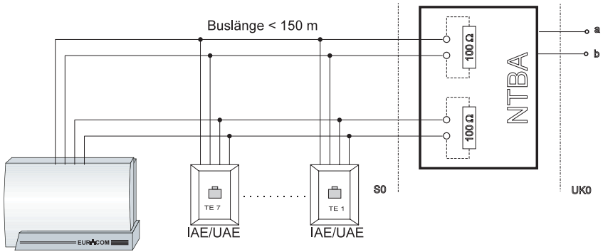
ISDN-Mehrgeräteanschluß – Punkt-zu-Mehrpunktanschluß
